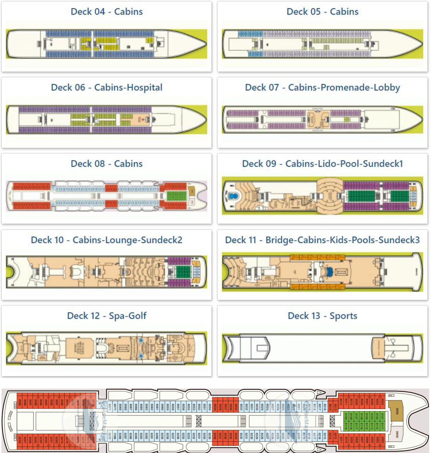
Resim 3 - Gemi Yerleşim Örneği
